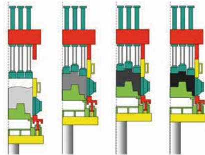
TWINPRESS kalıplama işleminin otomatik sırası Schematic sequence of the TWINPRESS moulding process
